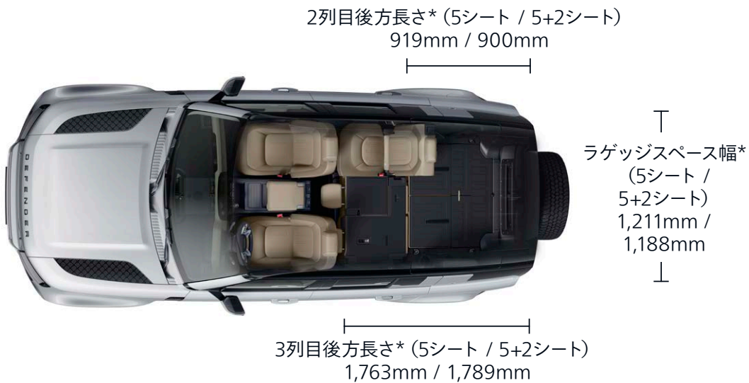
全長4,945mm (スペアホイール非装着時)
